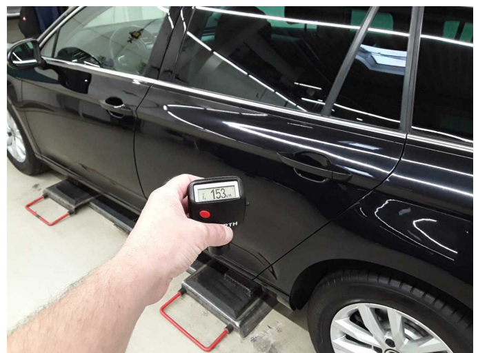
Door - rear left side: 153 \mu\text{m}
