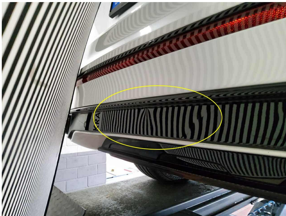
Bild 29 : Diffusor deformiert
