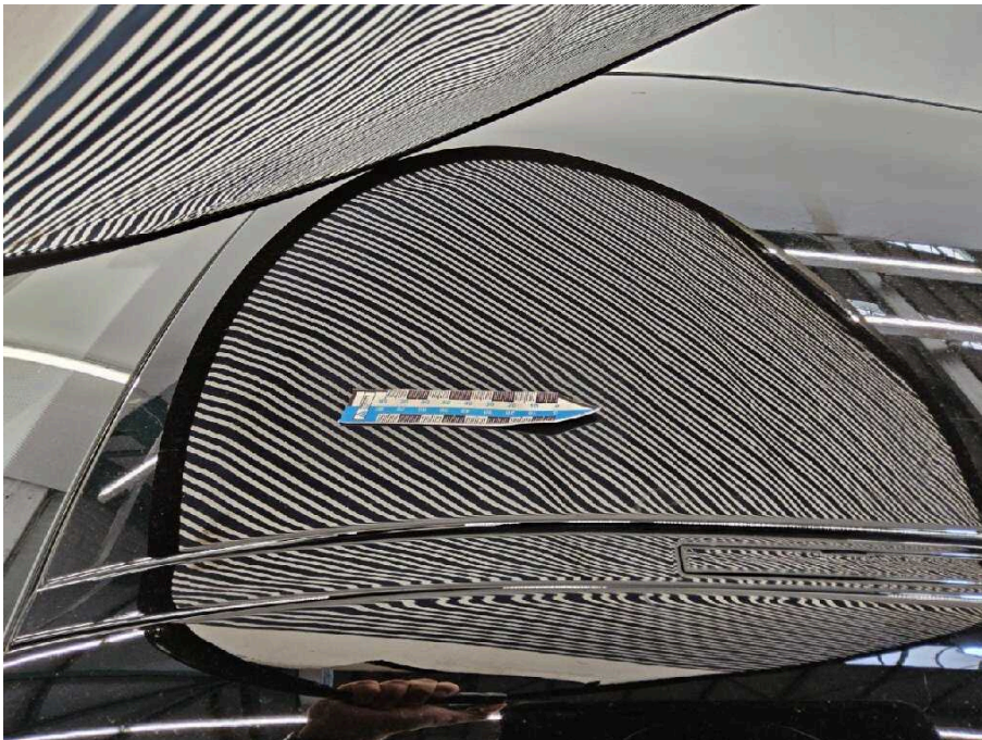
Bild 42 Dach Dachhaut deformiert
