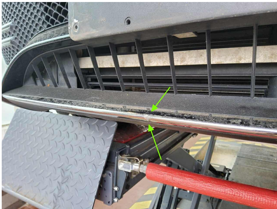
Bild 25 : Stoßfängerverkleidung vorn verschrammt und eingekerbt
