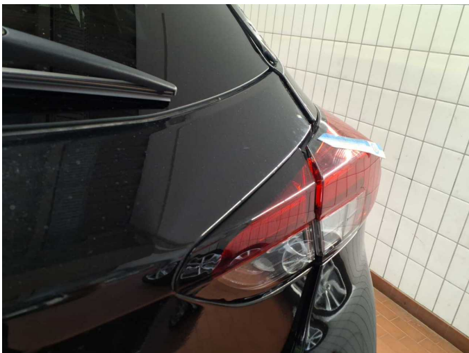
Damage 4: Boot lid / rear door: Boot lid (Spaltmaße) - Malposition - Set / adjust
