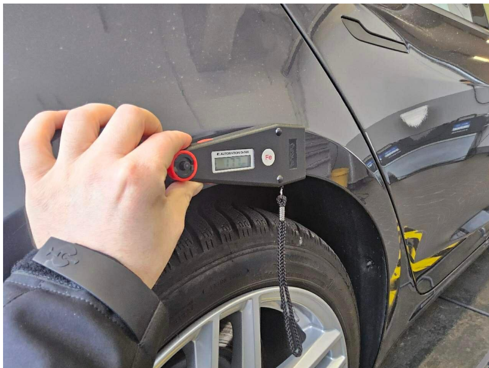
Bild 46 : Seitenwand hinten rechts, Lackschichtdicke 177 \mu m
